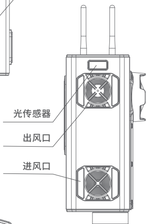
左视图
